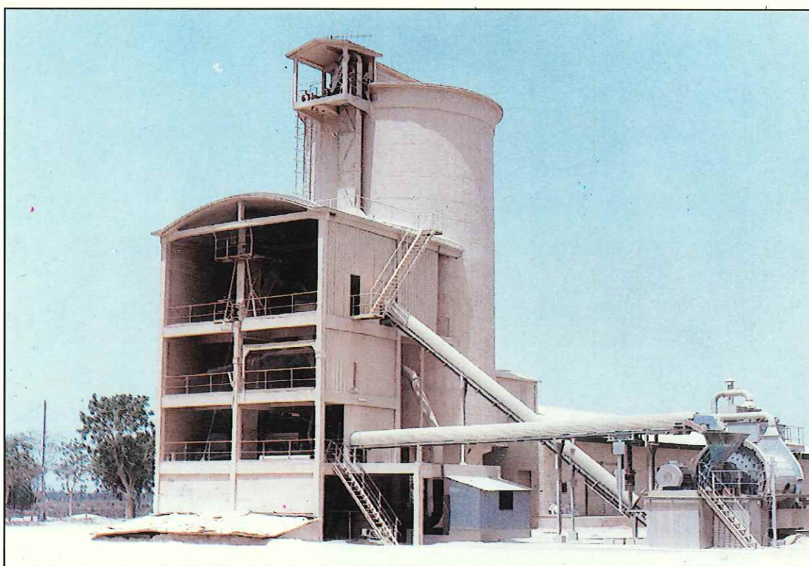
Phosphates de Thiès : broyage fin et silo de stockage - République du Sénégal.
